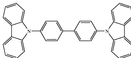
CBP
