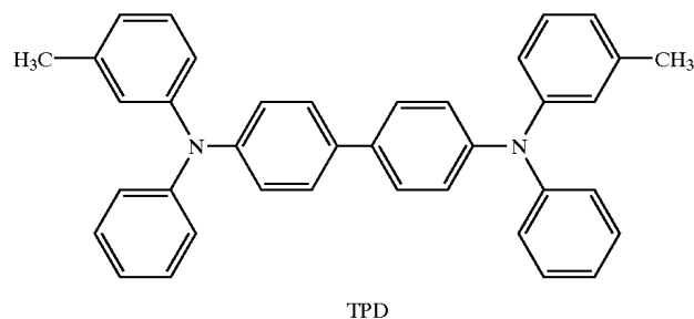
TPD
