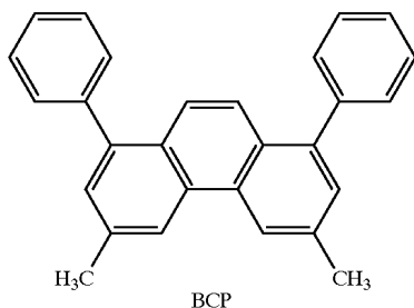
BCP
